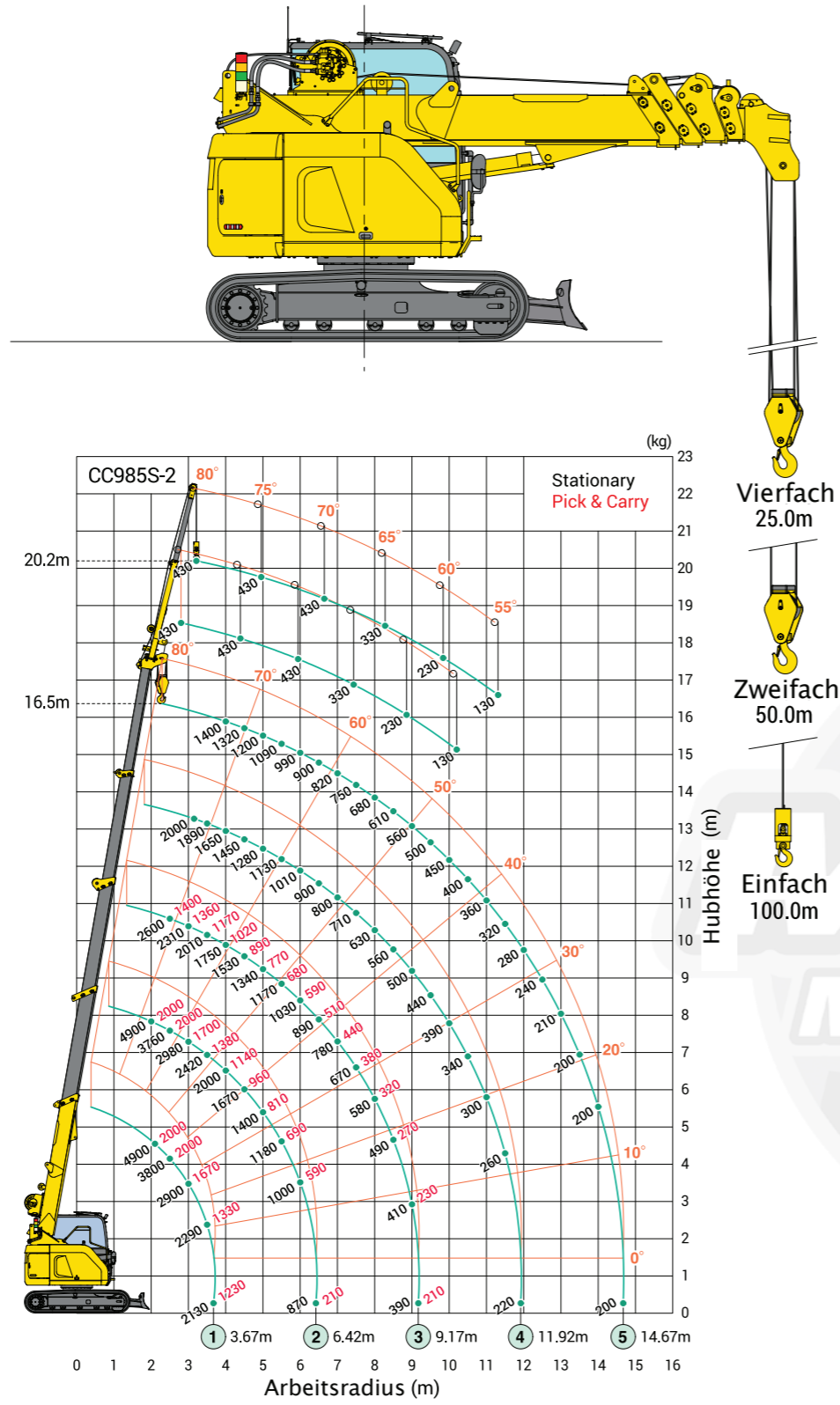
Das Arbeitsbereich-Diagramm zeigt die Gesamtlast einschließlich der Reichweite des Auslegers und der Fly Jib.
