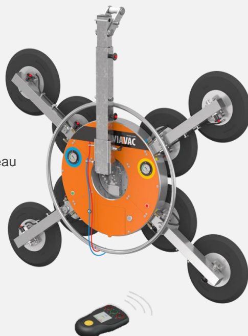
Optional Funkfernsteuerung
